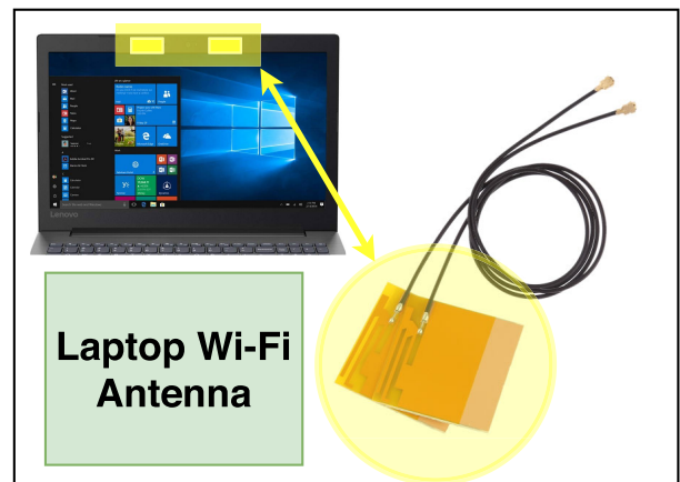
(d) Wi-Fi antennas in a laptop
